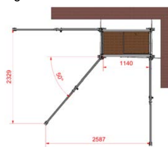
Montage der Wandabstützung
