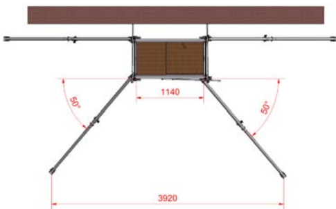
Montage der Wandabstützung
