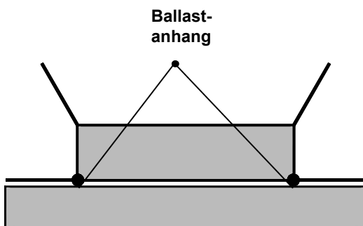
Abb.3 Ballastanhang bei Wandposition
